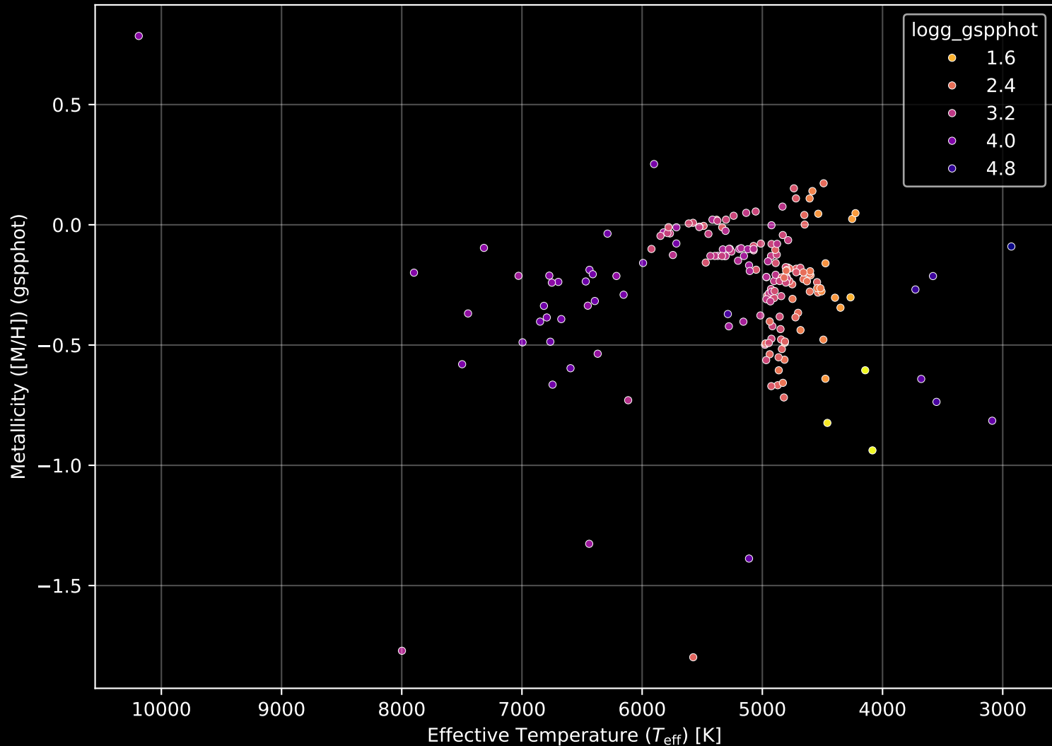
APOGEE DR17 Field: [180+30] Stellar Population Parameters (n= 193)
